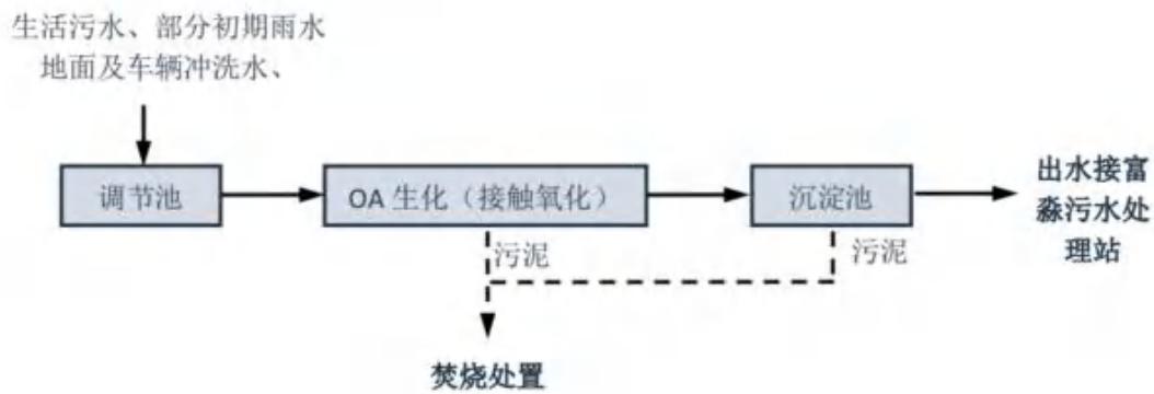
图4.1-1 综合污水一体化处理设备处理工艺流程图
