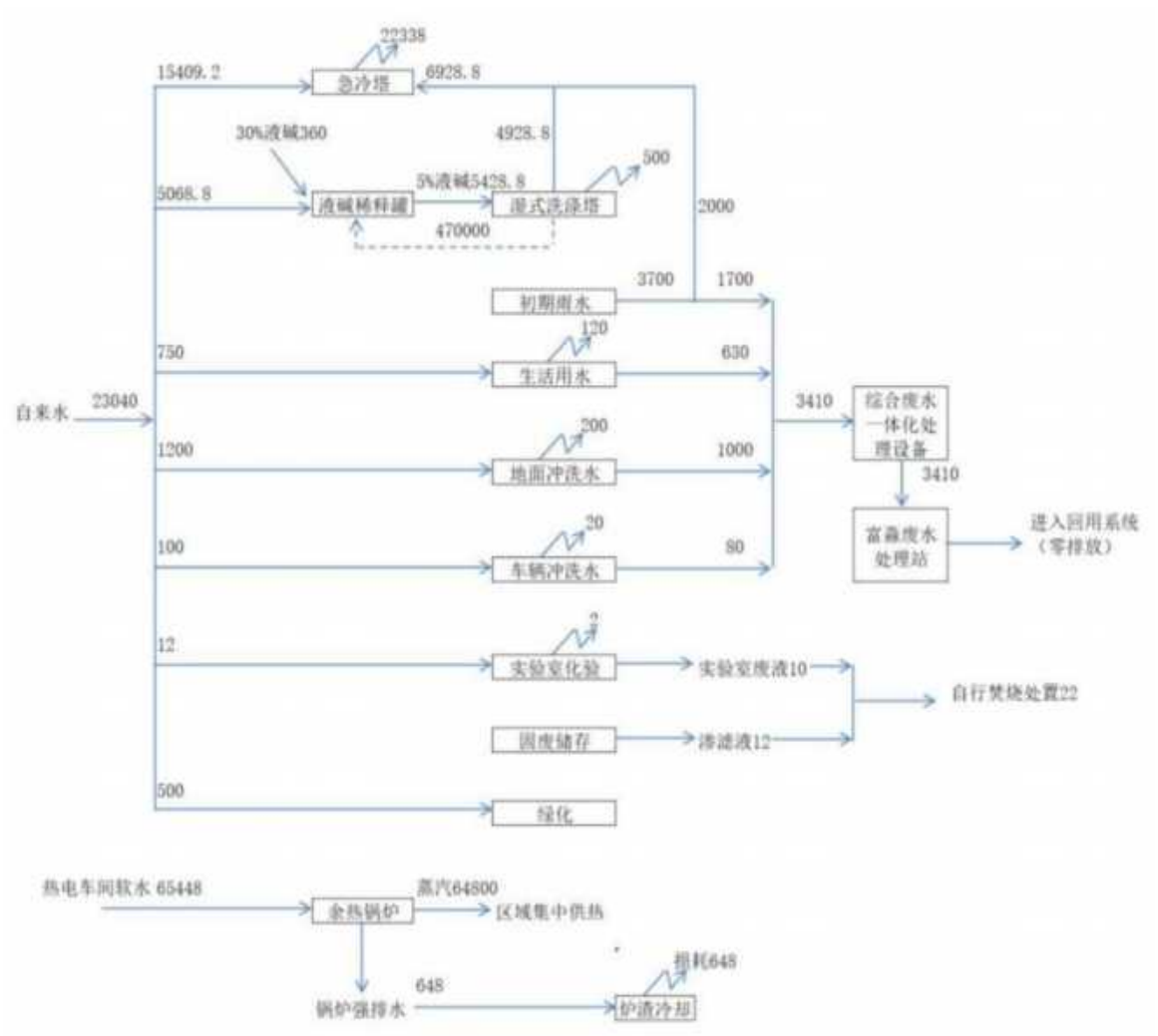
图3.4-1 本项目技改后全厂水平衡图 单位：t/a
