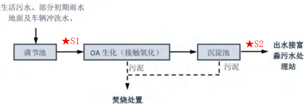
图 7.1-1 综合污水一体化处理设备采样点位图
