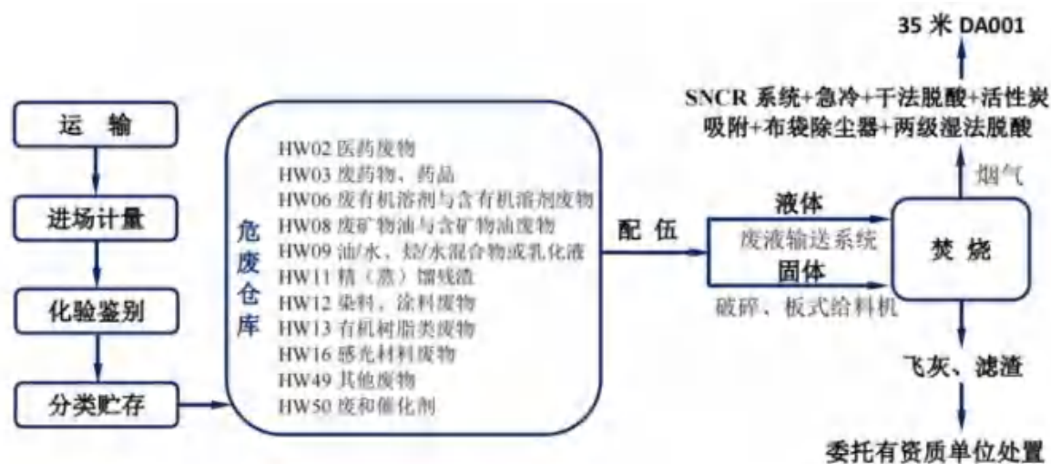
图3.5-1 总体工艺流程示意图
