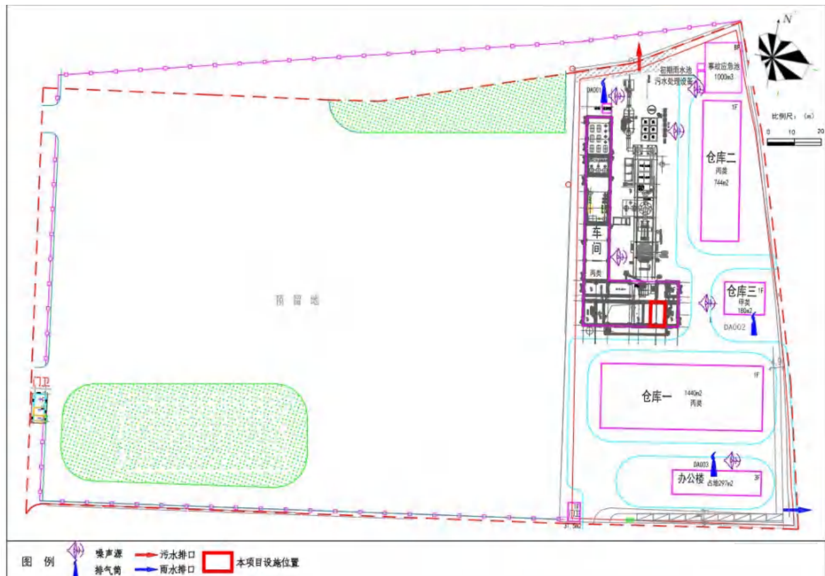
图3.1-3 项目厂区平面布置
