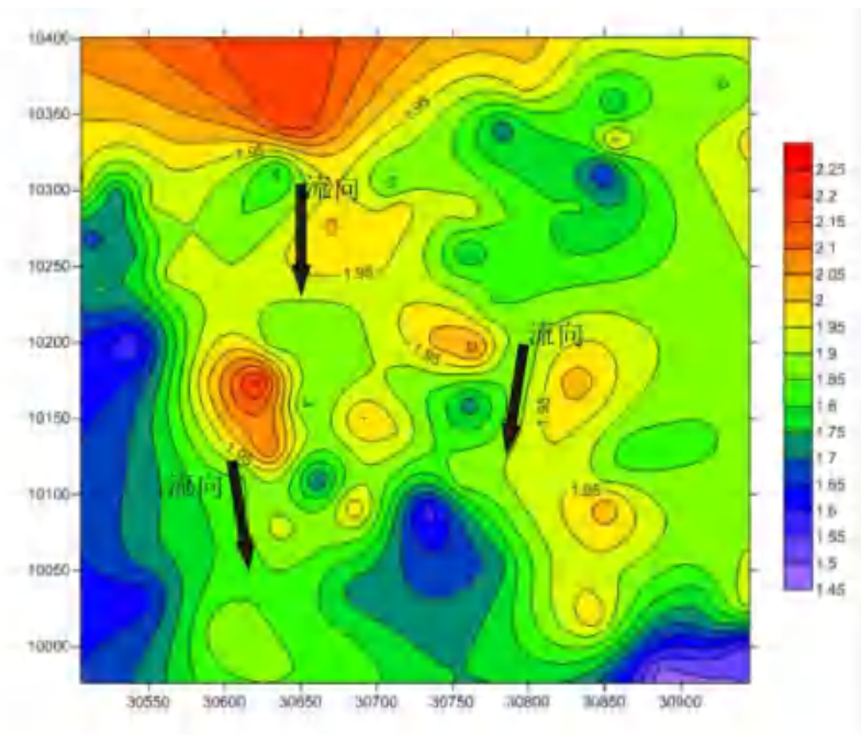
图 3.1-3 地下水位等高线及地下水流向图
