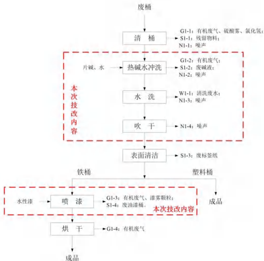
图3.3.1-1 本项目废包装桶清洗加工工艺流程图
