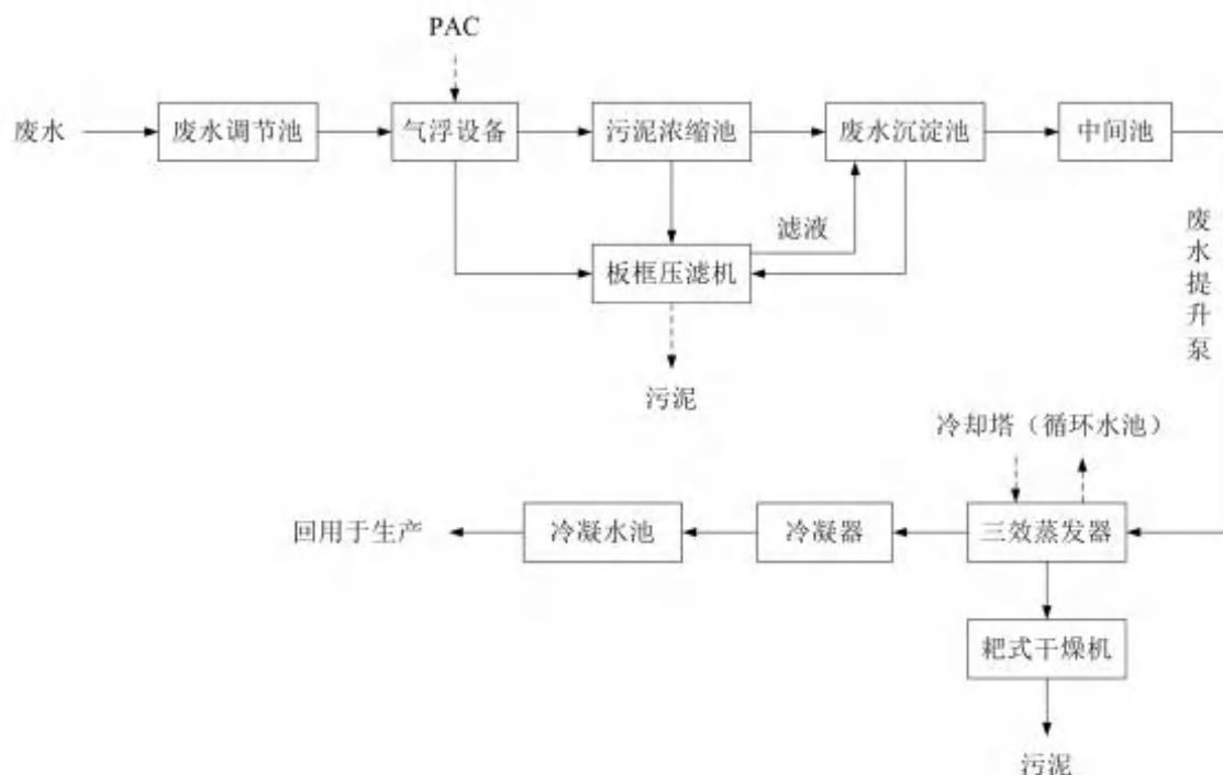
图4-1 废水处理流程图
