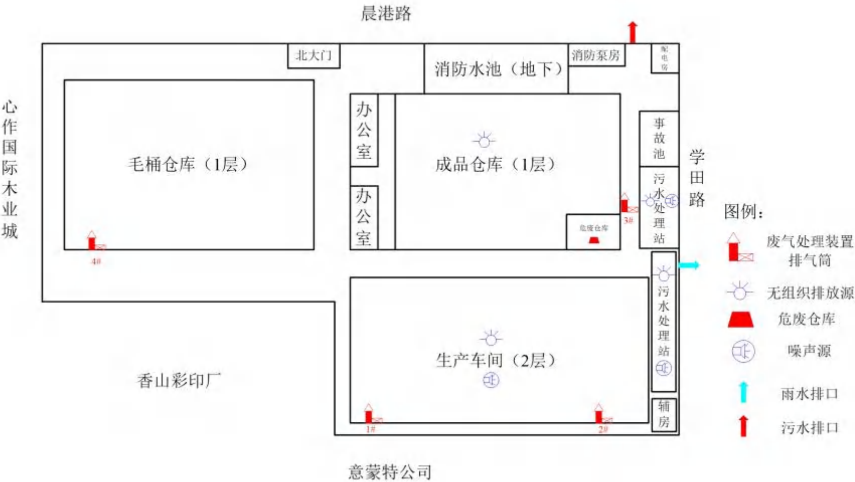
图3-3 环评设计平面布置图
