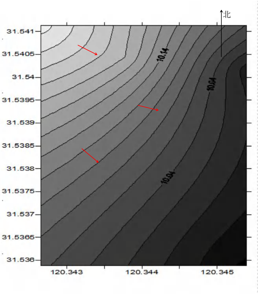
图 4.4-3 地块地下水流向图
